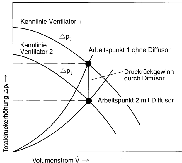
Bild 2: Druckrückgewinnung
