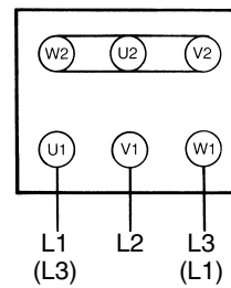
Y-kytkentä (korkeampi jännite)
