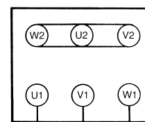
L1 L2 L3 (L3) (L1) Conexión en estrella (alta tensión)
