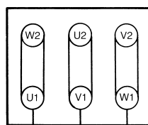
Δ-tilslutning (lav spænding)
