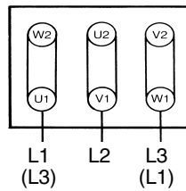
Circuito \Delta (bassa tensione)
