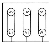
L1 L2 L3 (L3) (L1) Conexión de triángulo (baja tensión)
