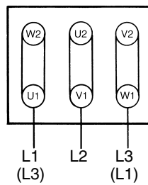
Δ-kytkentä (matalampi jännite)
